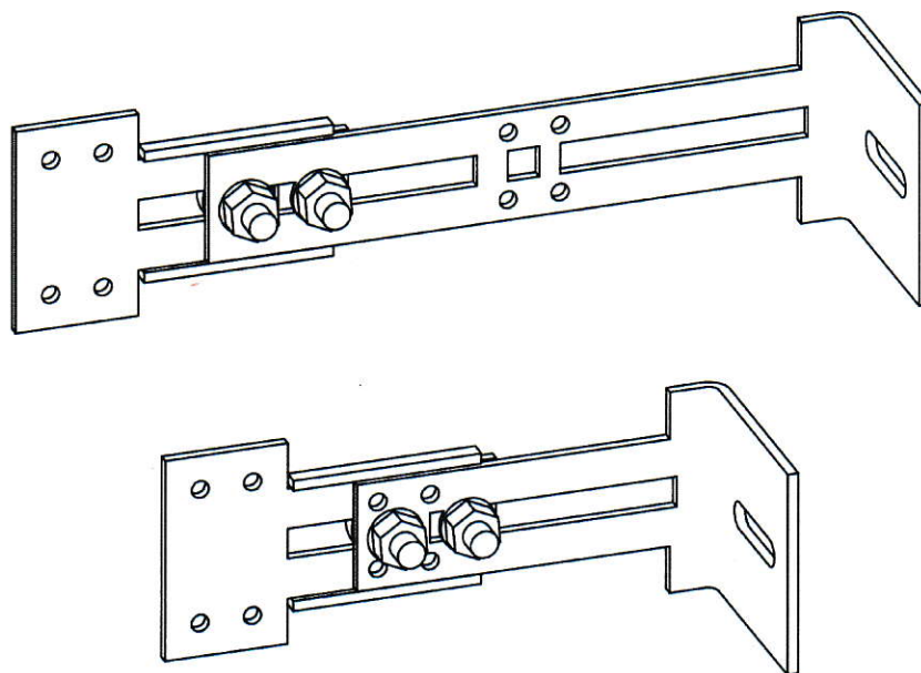
Rys. 3. Widok izometryczny złożeń analizowanych konsol przy maksymalnych wsięgach (z uwagi na geometrię).
