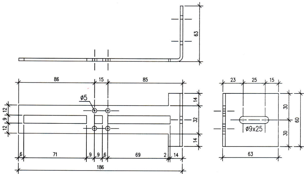
Rys. 5. Wymiary wspornika – część stosowana w konsoli: Typ A.
