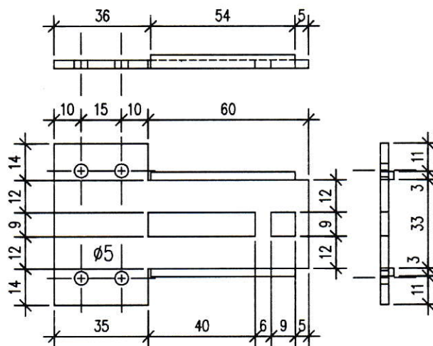
Rys. 6. Wymiary blachy złącznej – część stosowana w konsolach: Typ A i Typ B.
