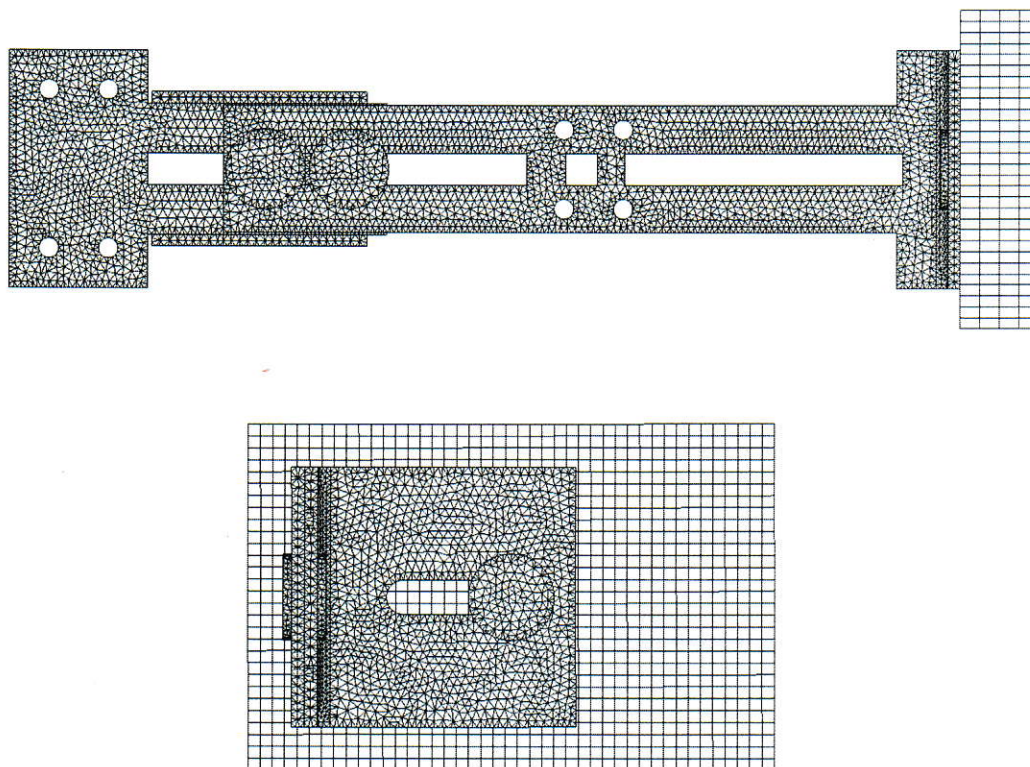
Rys. 7. Model obliczeniowy konsol z wykonanym siatkowaniem.
