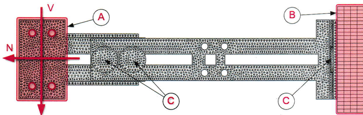
Rys. 8. Warunki brzegowe – schemat ogólny (opis w tekście).
