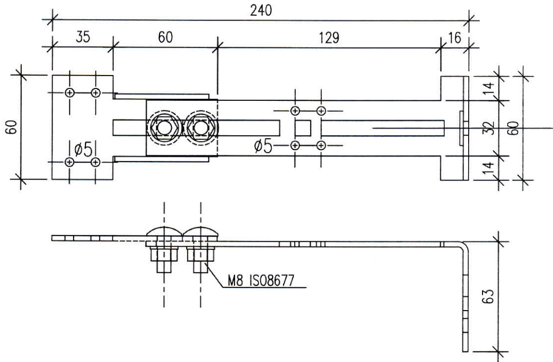
Rys. 4. Wymiary orientacyjne przy maksymalnym wysięgu konsoli – Typ A.
